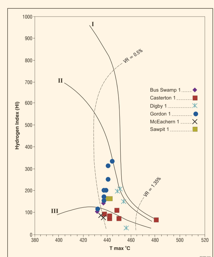
HI vs Tmax plt, Casterton Formation
